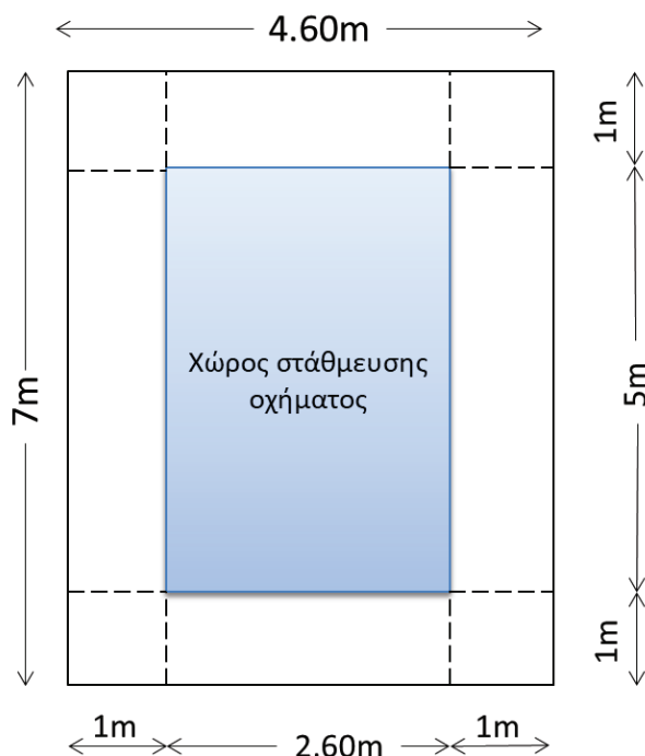
Εικόνα 1:Σκαρίφημα χώρου αναμονής και ελέγχου οχημάτων υψηλής τάσης
